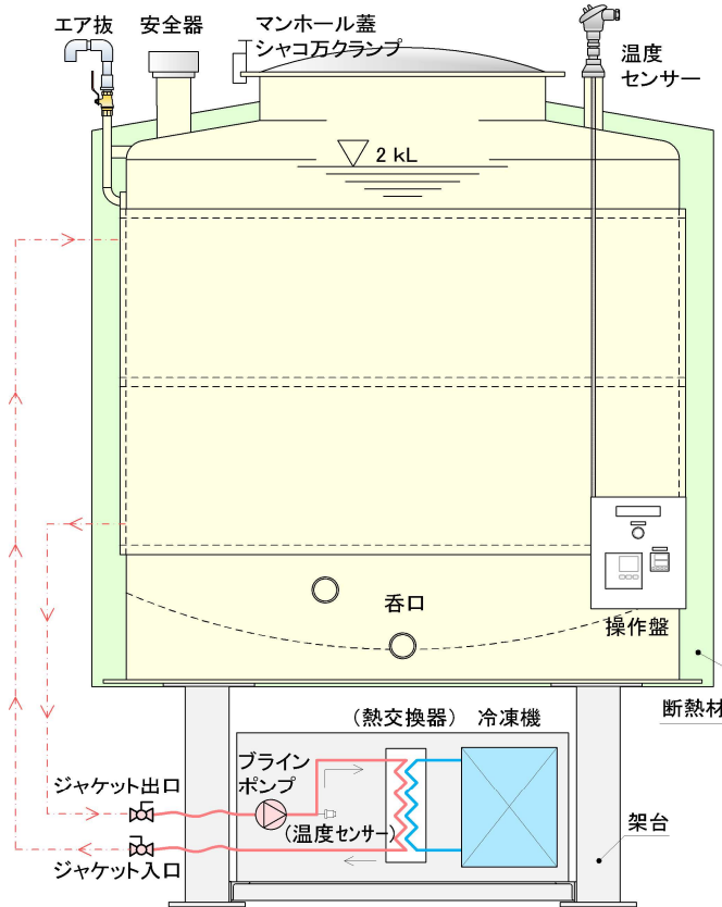
2000Lクーリングタンク(標準型)
